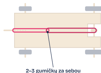
Pohled shora: gumička od háčku po kartonu na zarážku, ani volná, ani napnutá
